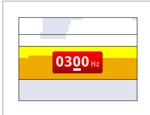
Figura 28 – Alterar tom
